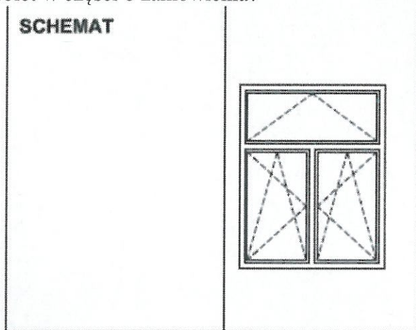
Rysunek 1 Okno o wymiarach szer. 160 wys. 200
