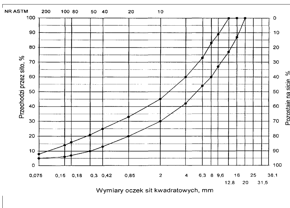
Rys. 6. Krzywe graniczne uziarnienia mieszanki mineralnej BA od 0 do 16 mm do warstwy wyrównawczej nawierzchni drogi o obciążeniu ruchem od KR3 do KR6
